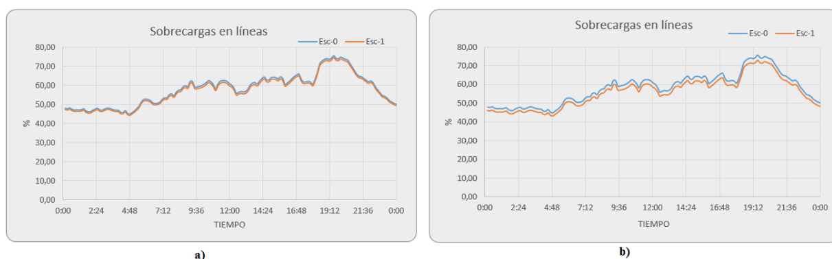
Figura 7. Sobrecargas en las líneas: (a) micro-red normal, b) micro-red x10.
