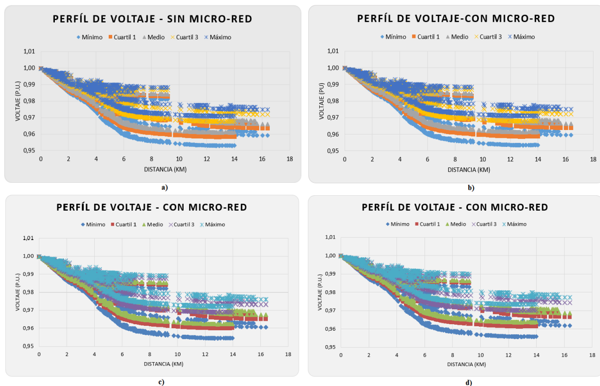
Figura 6. Perfil de voltaje. a) Sin micro-red, b) Con micro-red normal, c) Con micro-red x5, y d) Con micro-red x10.
