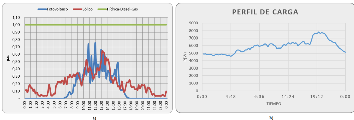
Figura 4. a) Perfil de generación, b) Perfil de carga del alimentador.
