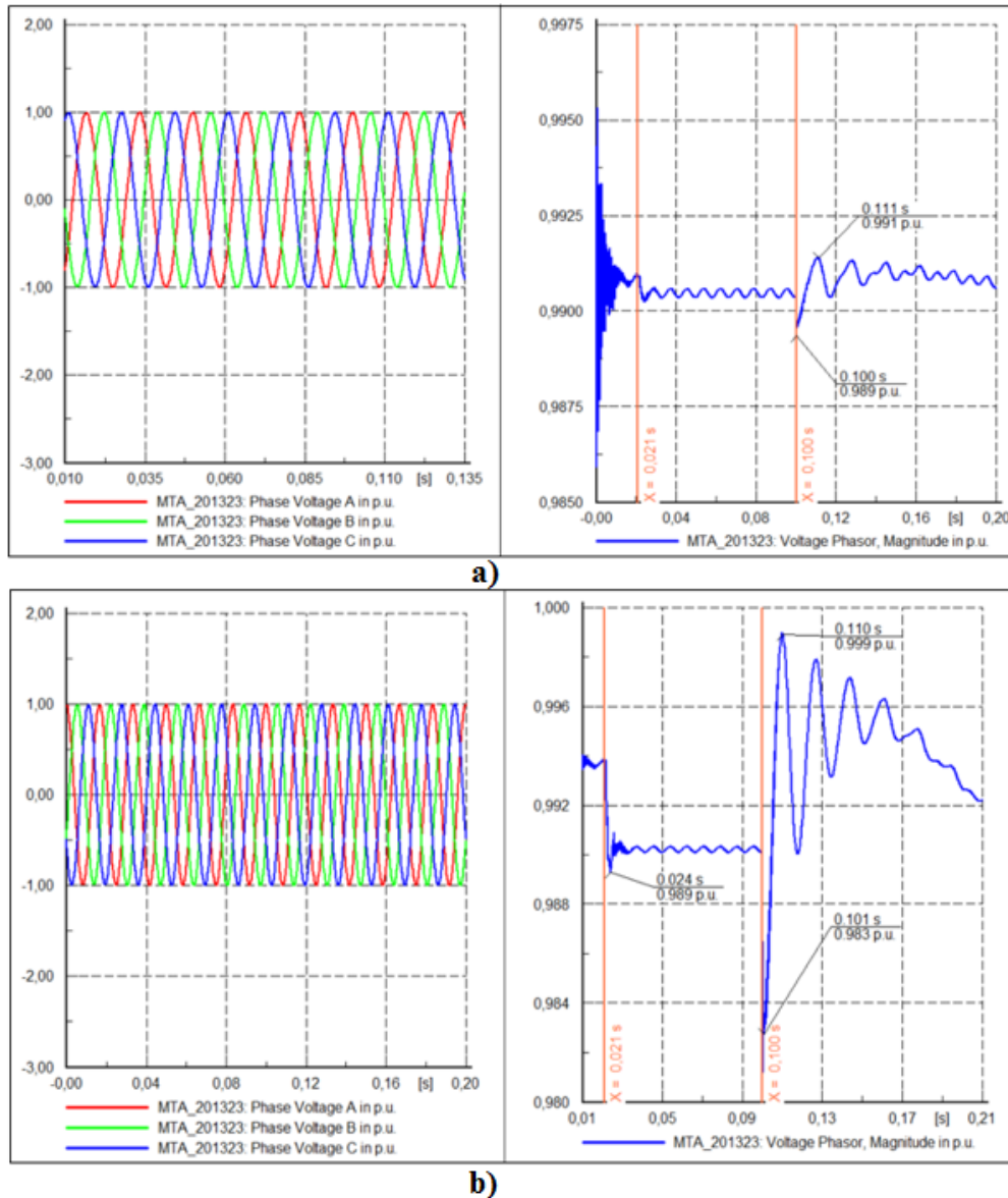
Figura 8. Sobrevoltajes (p.u.) en el PCC luego del evento desconexión/conexión de la micro-red normal; a) micro-red normal, b) micro-red x10.
