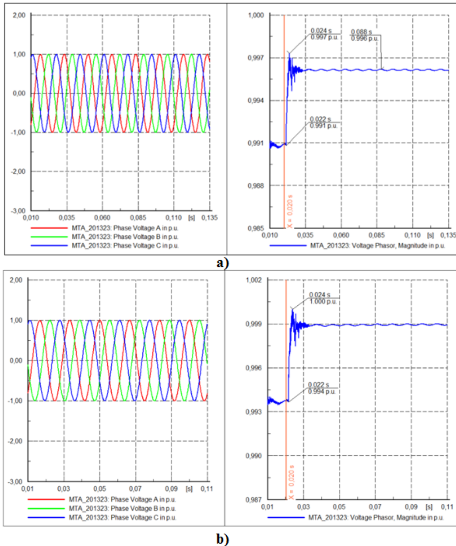
Figura 9. Sobrevoltajes (p.u.) en el PCC luego del evento de “switch” (abre reconector R1); a) micro-red normal, b) micro-red x10.
