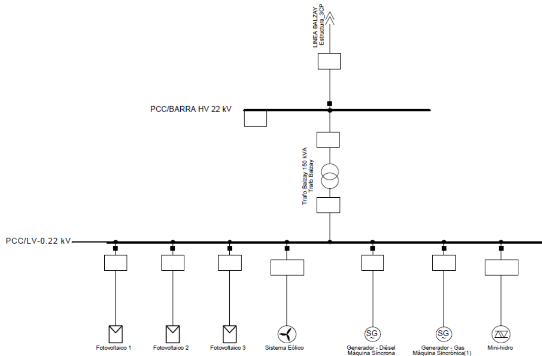
Figura 3. Esquema unifilar de la micro-red conectado a la red de distribución.
