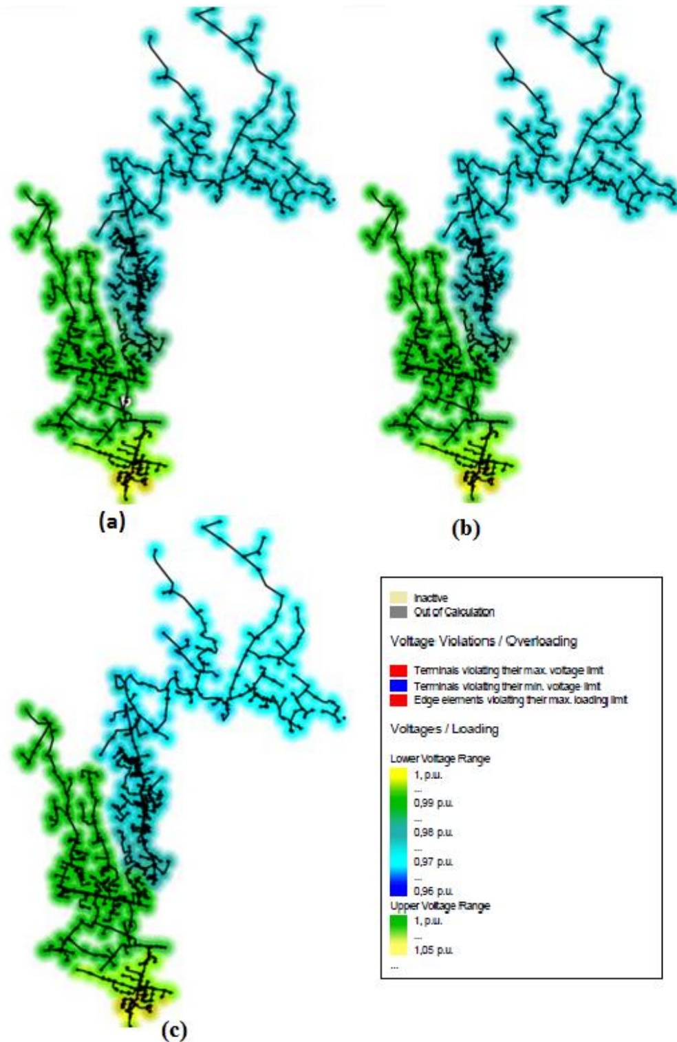
Figura 5. Mapa de calor de voltajes en p.u. en los nodos del alimentador 0523, (a) Escenario “0”, sin Micro-red, (b) Caso 1s conectado micro-red normal, (c) Caso 1s conectado micro-red x 10.
