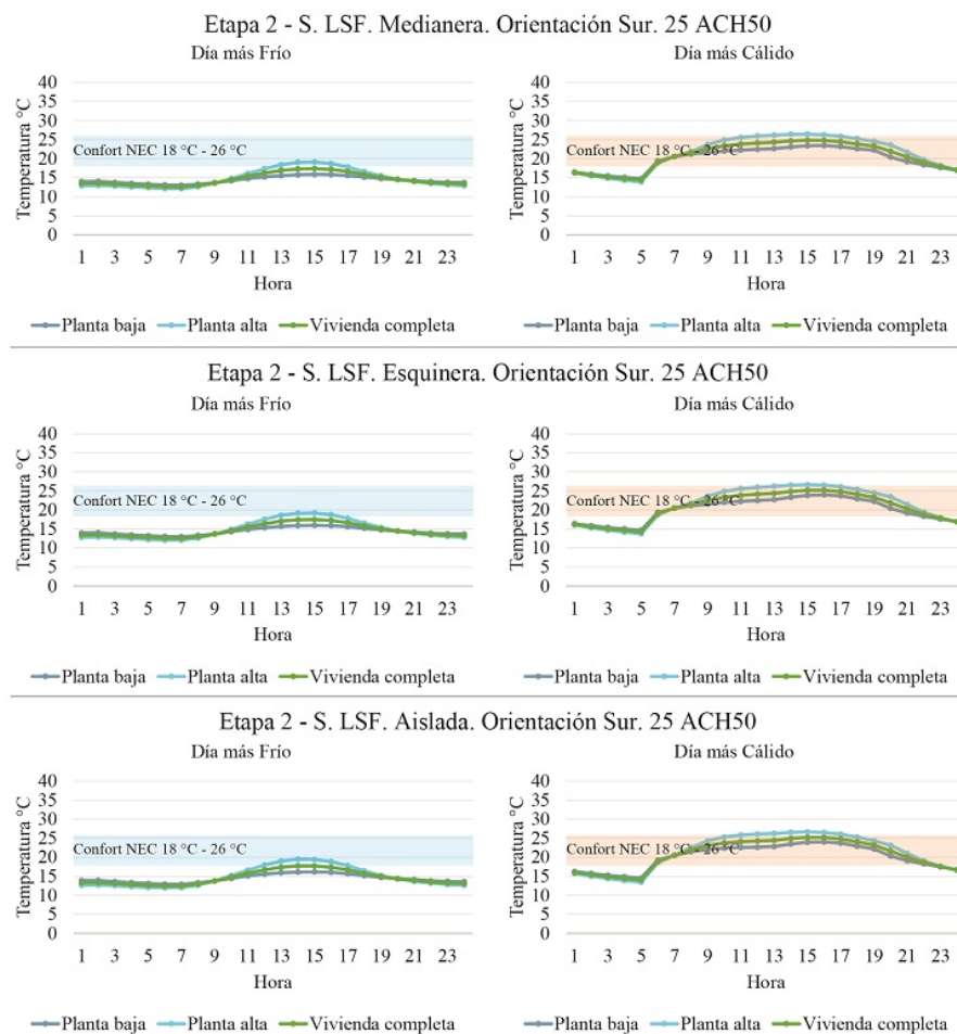
Figura 9. Comparativa térmica, sistema LSF, segunda etapa
