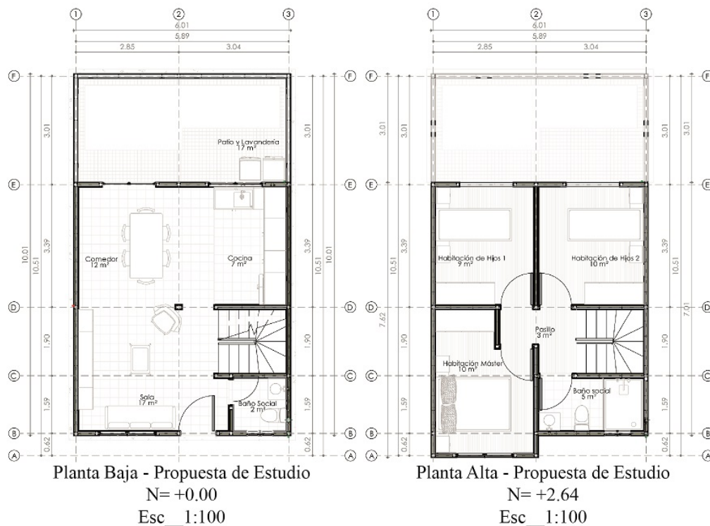
Figura 5. Propuesta materializada con LSF
