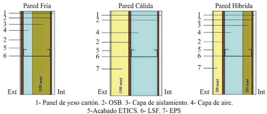
Figura 11. Tipologías de pared: cálida, fría e híbrida
