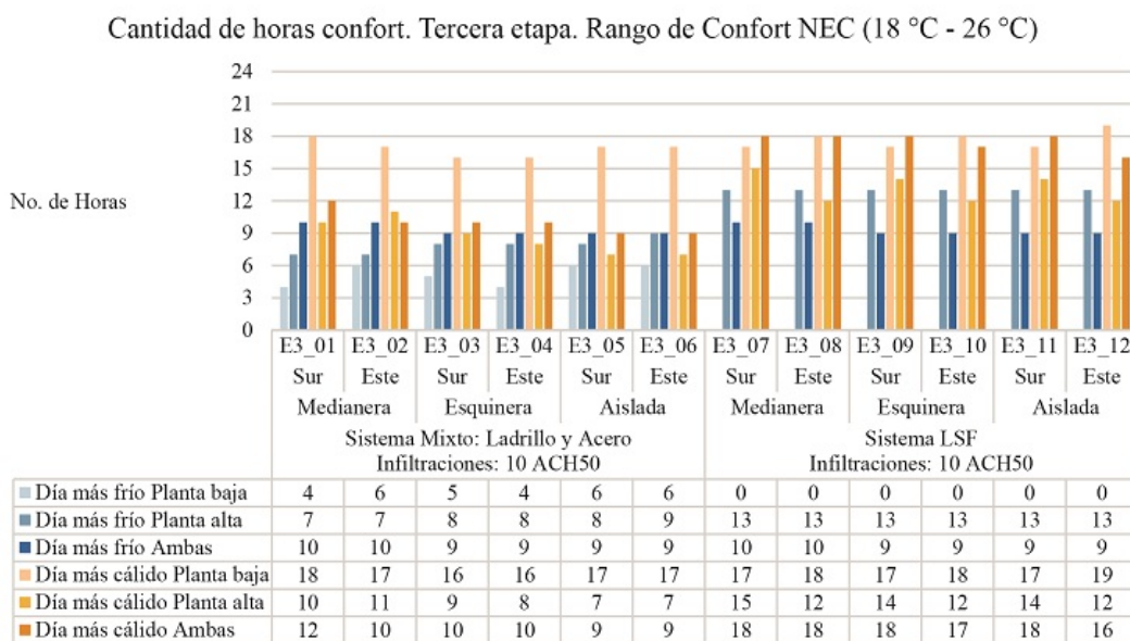
Figura 15. Comparativa del número de horas confort de la tercera etapa
