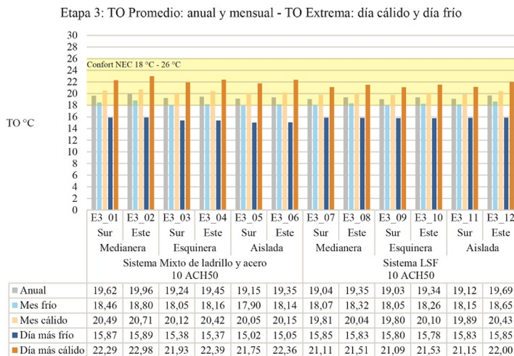
Figura 14. Comparativa térmica general de la tercera etapa
