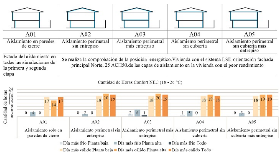
Figura 12. Tipos de aislamiento y rendimiento energético en número de horas confort
