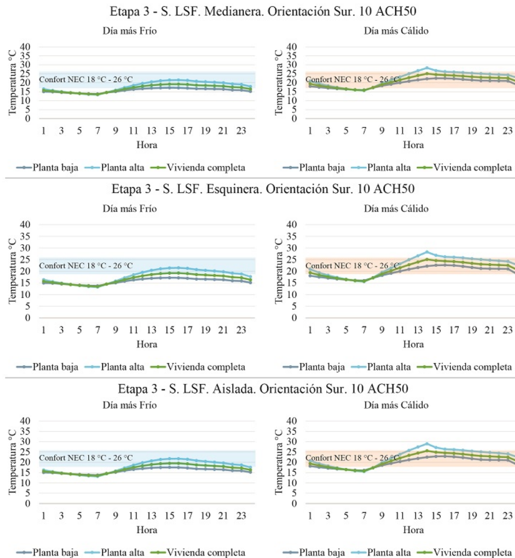
Figura 17. Comparativa térmica, sistema LSF, tercera etapa
