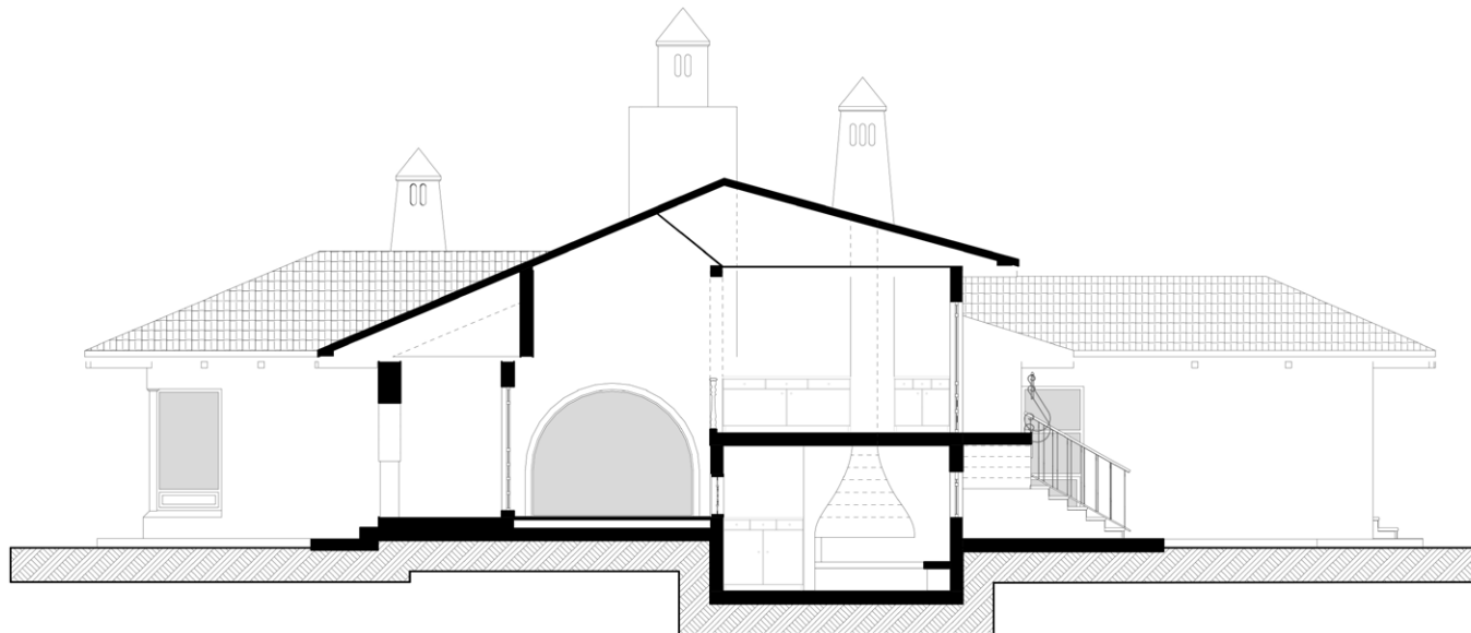
Fig. 082 Redibujo documentación Vivienda Salazar Harris
