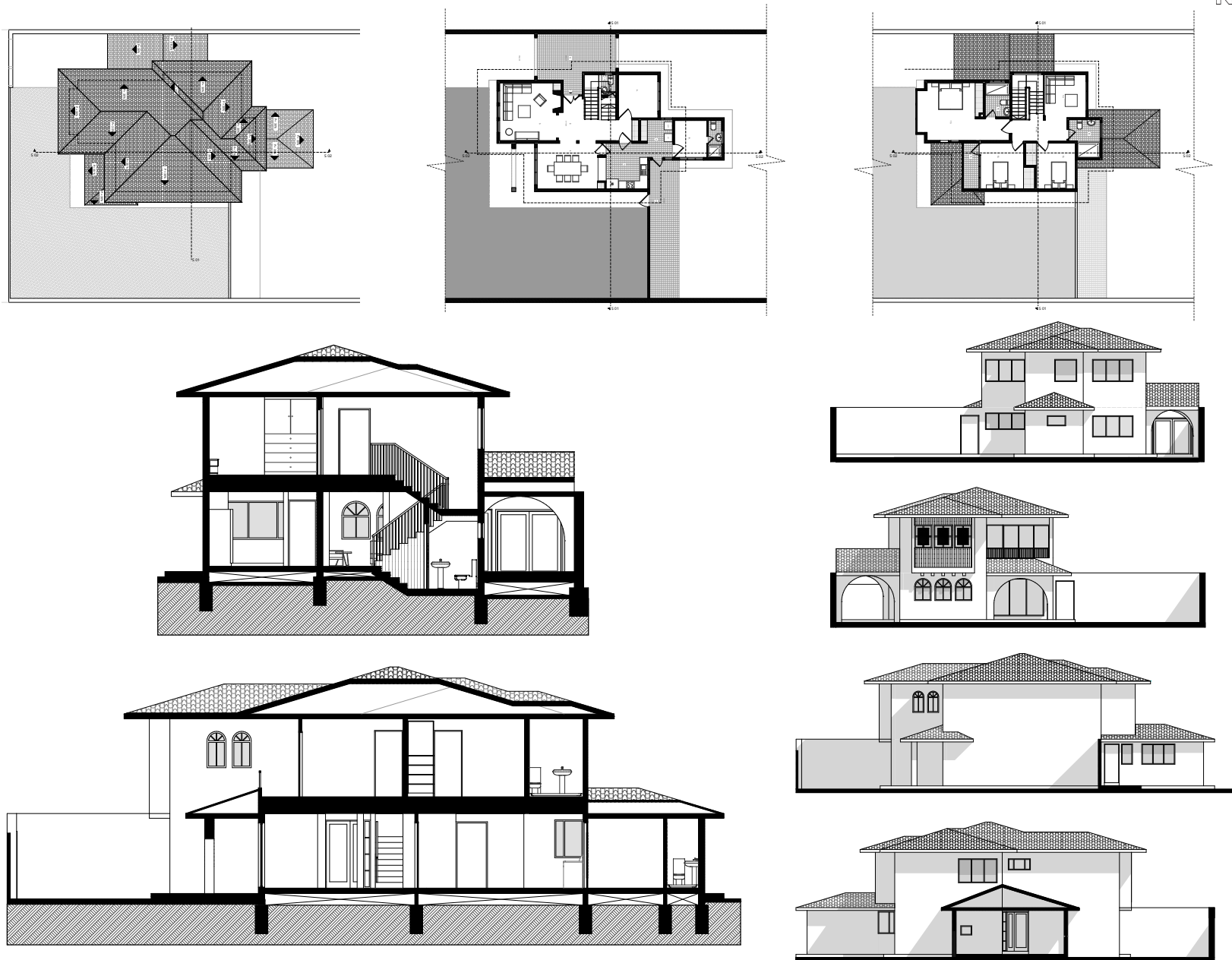
Fig. 094 Redibujo documentación Vivienda María Elena Serrano
