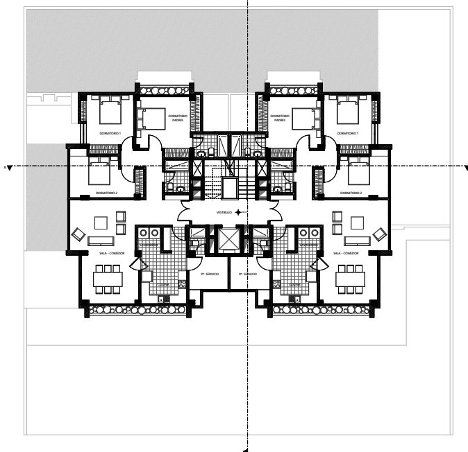
Fig. 156 Redibujo documentación edificio Los Álamos
