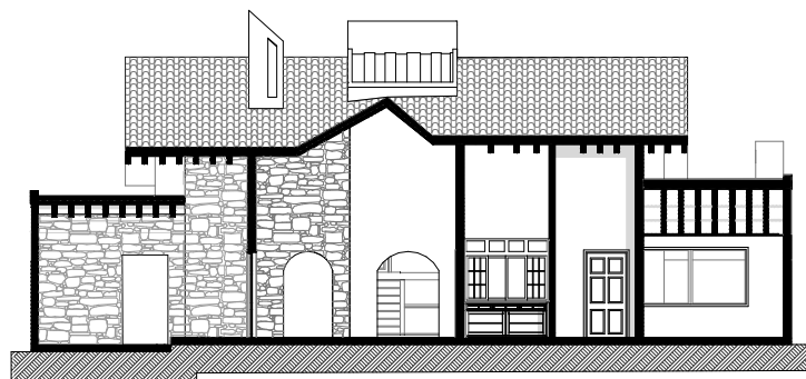
Fig. 124 Redibujo documentación vivienda Antonio Torres
