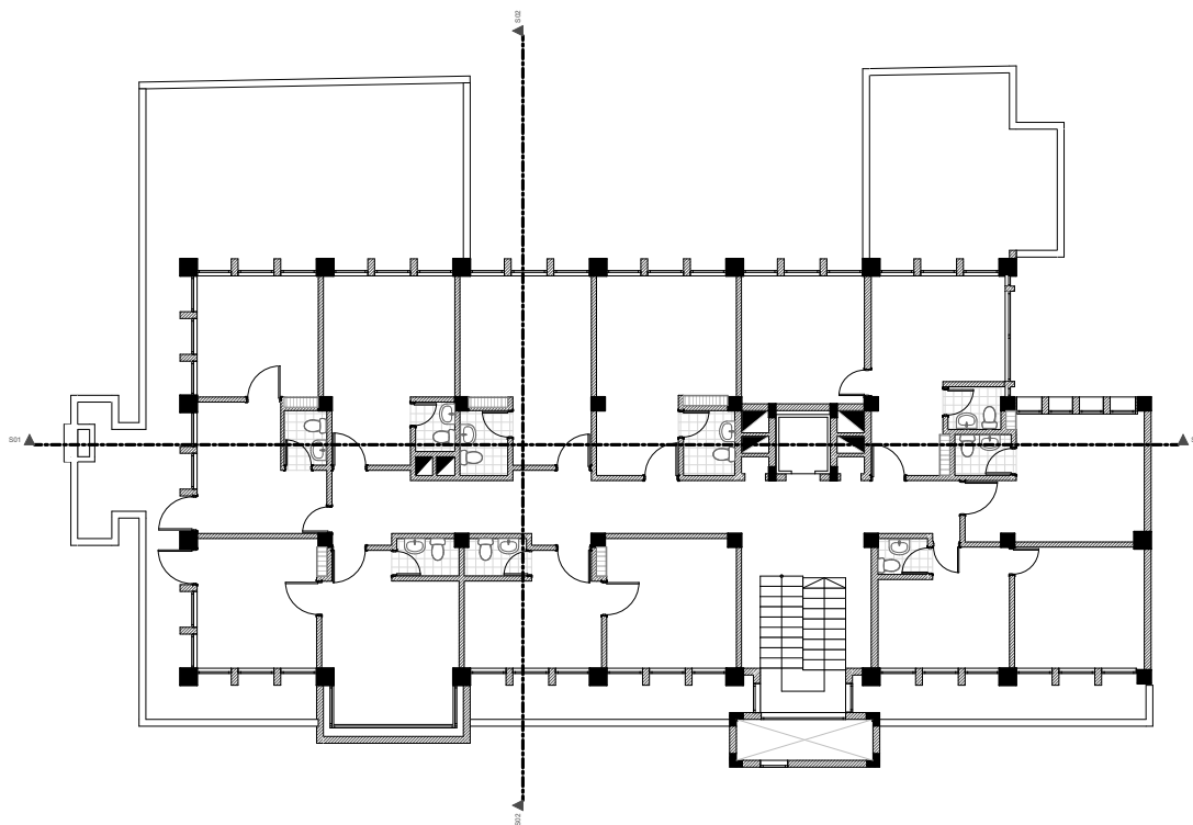
Fig. 130 Redibujo documentación Edificio COVAG II
