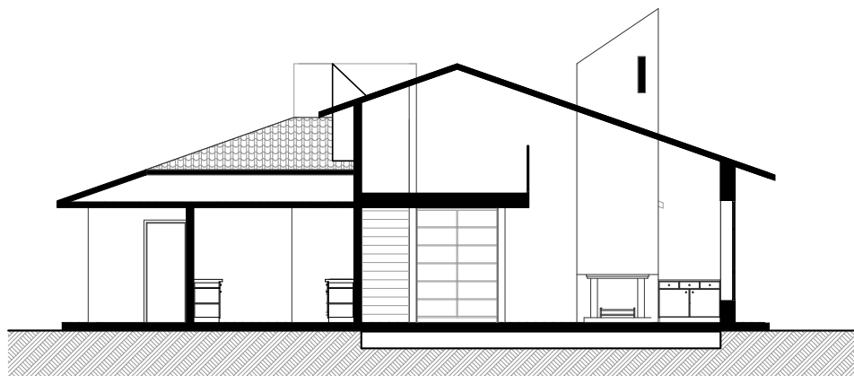
Fig. 169 Redibujo documentación vivienda Fabiola Arízaga
