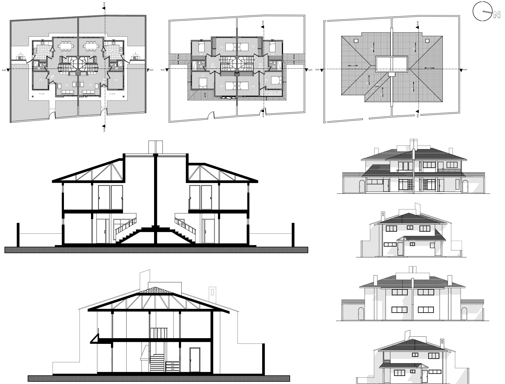
Fig. 068 Redibujo documentación Viviendas Emilio Isaías Lotes 3 - 6
