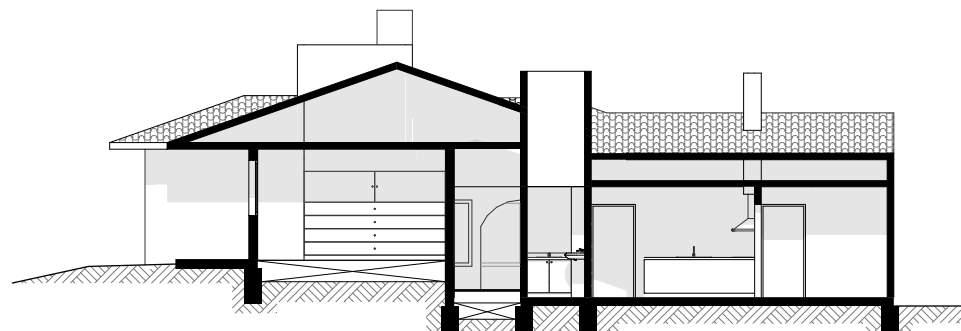
Fig. 106 Redibujo documentación Vivienda Marco Carrión
