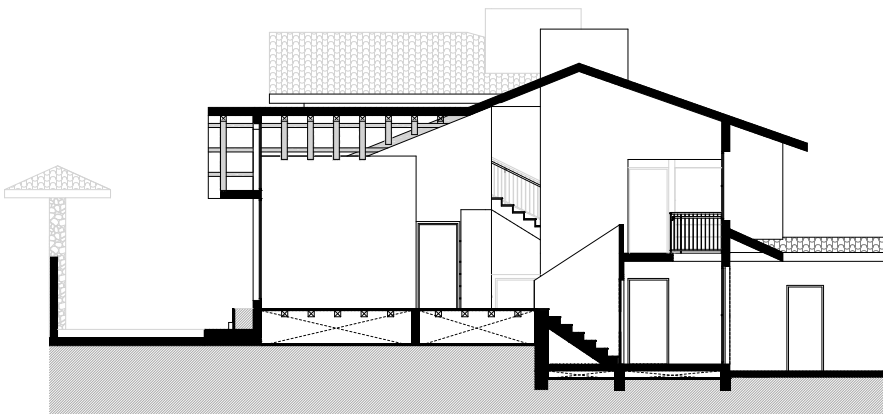
Fig. 127 Redibujo documentación vivienda Leonel Ugalde
