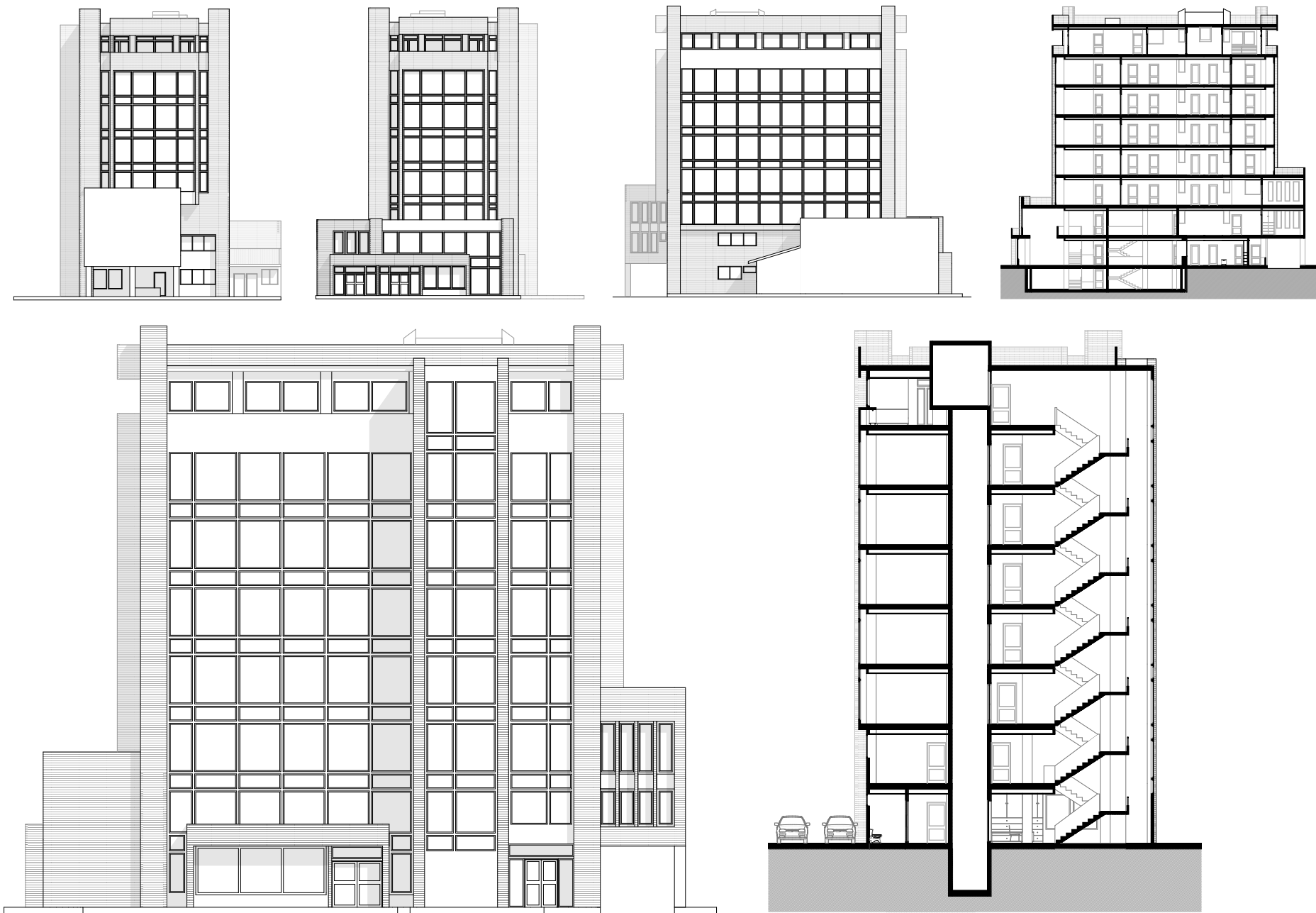
Fig. 163 Redibujo documentación edificio El Profesional
