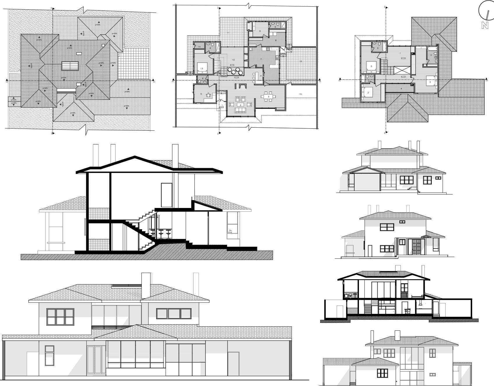
Fig. 097 Redibujo documentación Vivienda Jaime Torres
