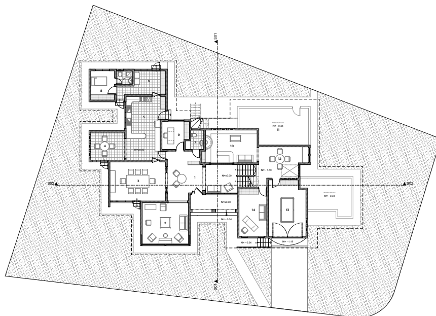
Fig. 076 Redibujo documentación Vivienda Salazar Harris
