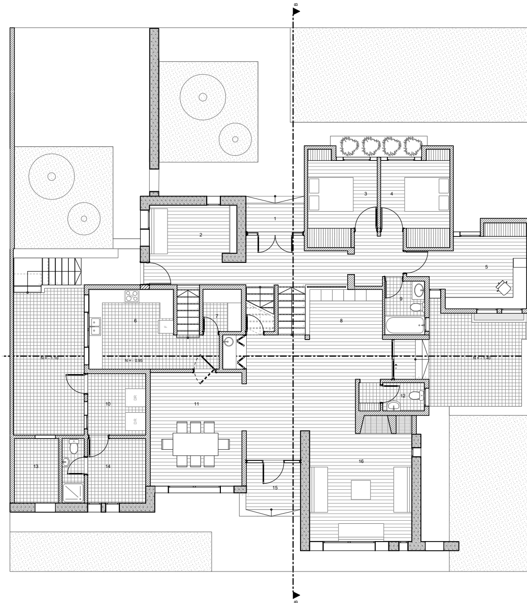
Fig. 138 Redibujo documentación vivienda Jail Díaz
