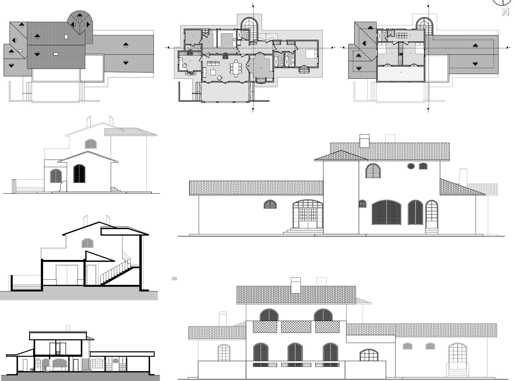
Fig. 073 Redibujo documentación Vivienda Luis Jaramillo
