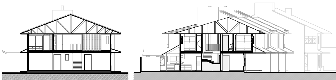
Fig. 150 Redibujo documentación Complejo Habitacional Huaynacápac
