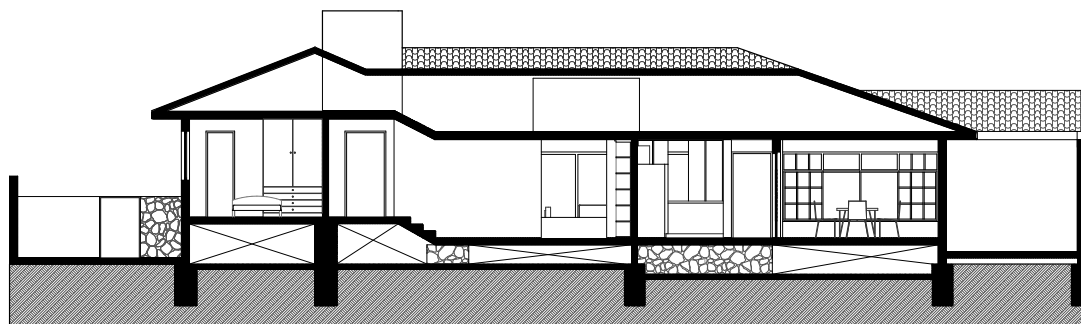
Fig. 100 Redibujo documentación Vivienda Pedro Cueva
