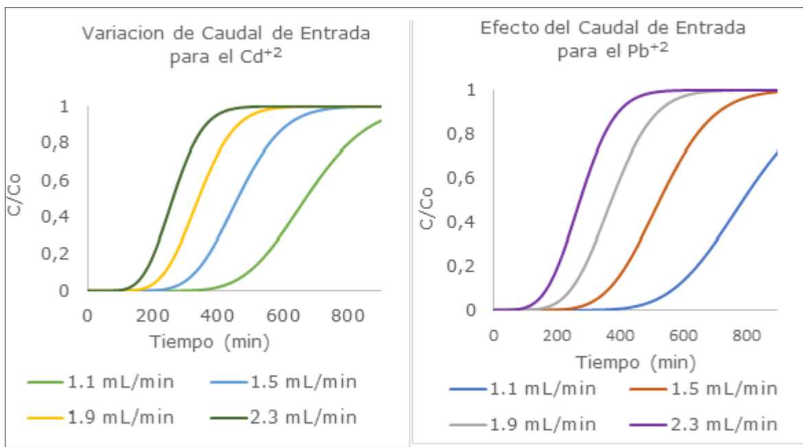
Figura 4 (a) y (b). Curva de ruptura para \text{Cd}^{+2} y \text{Pb}^{+2} variando el caudal de alimentación con una altura de lecho de 10.5 cm, 10 mg/L de Co y 18°C.
