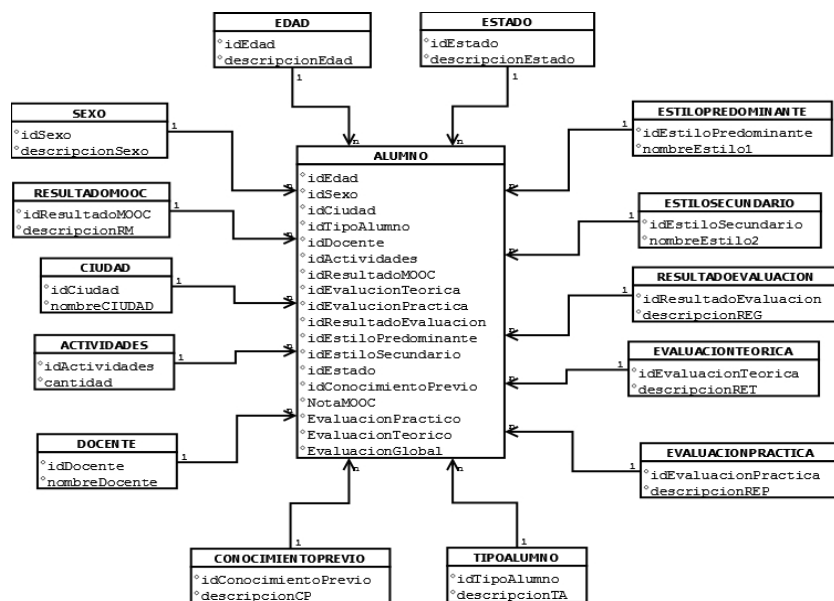
Figura. 2. Modelo lógico estrella para la construcción de un datawarehouse
