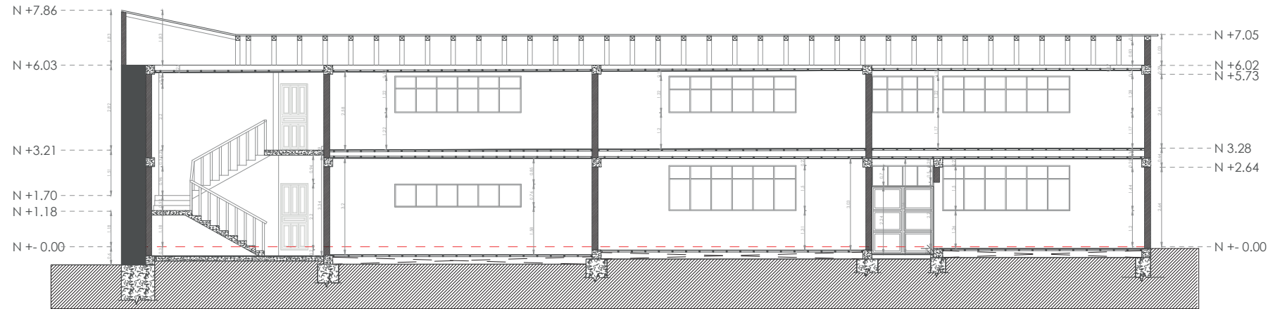
CORTE E-E ESTADO ACTUAL
