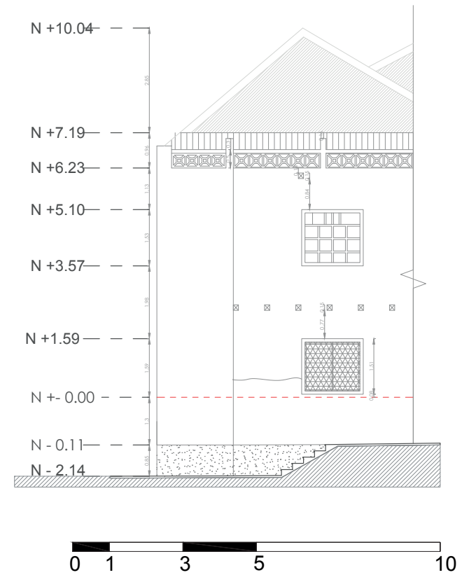
Fig 179: Redibujo, alzado lateral derecho estado actual
