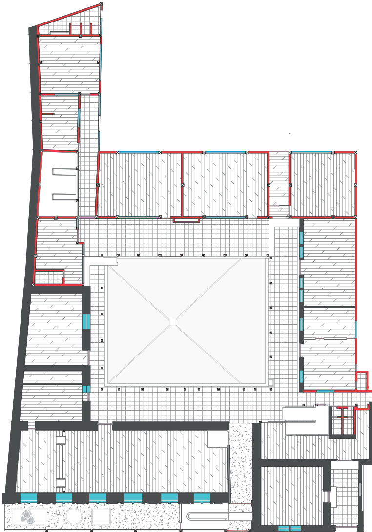
Fig 187: Materialidad Planta Baja Pisos, paredes, puertas y ventanas
