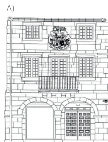
Fig 174: Planimetría de fachadas
