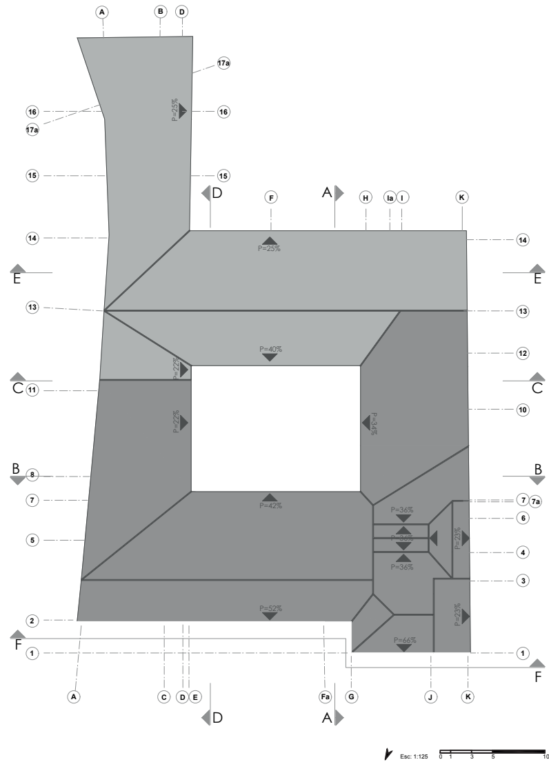
Fig 178: Redibujo, planta de cubiertas estado actual
