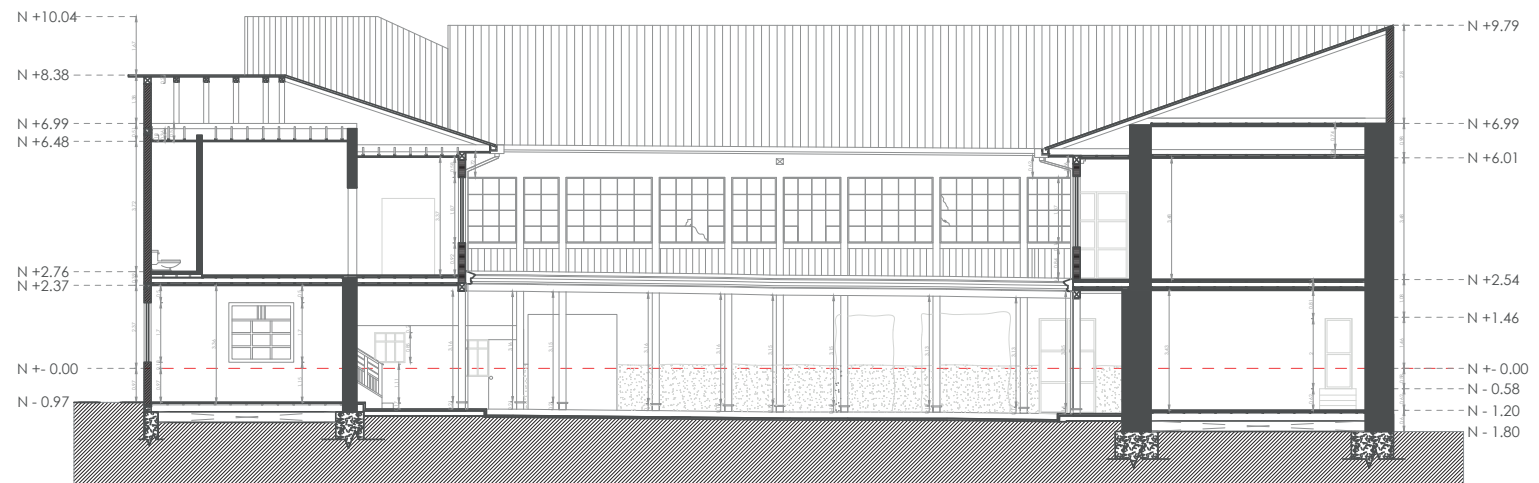
Fig 182: Redibujo, Corte A-A y B-B
