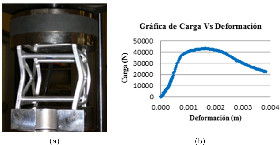
Figura 3. (a) Prueba destructiva; (b) Gráfica del ensayo.
