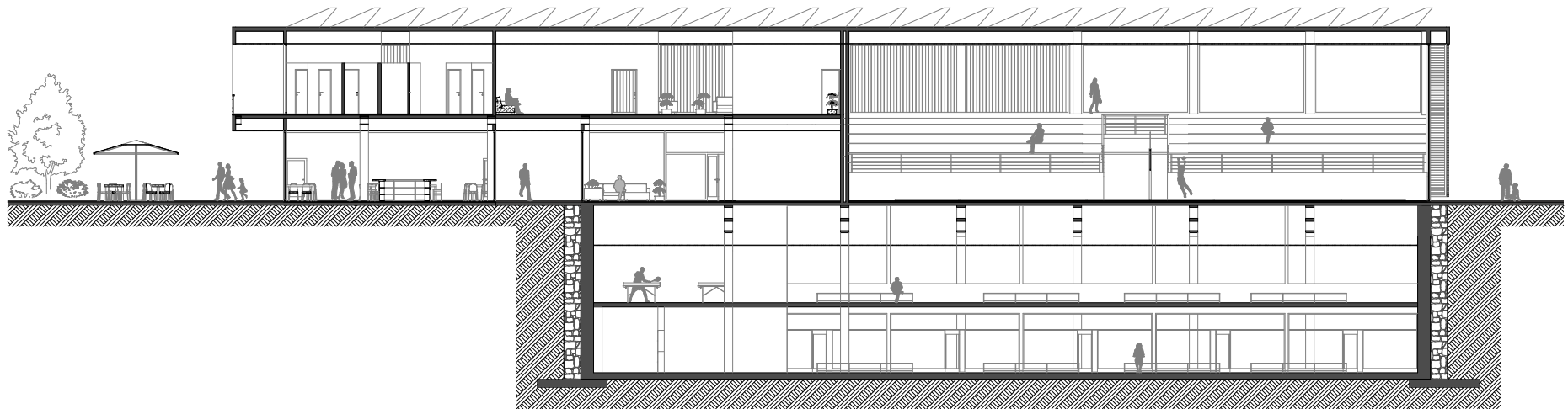
CORTE B-B
