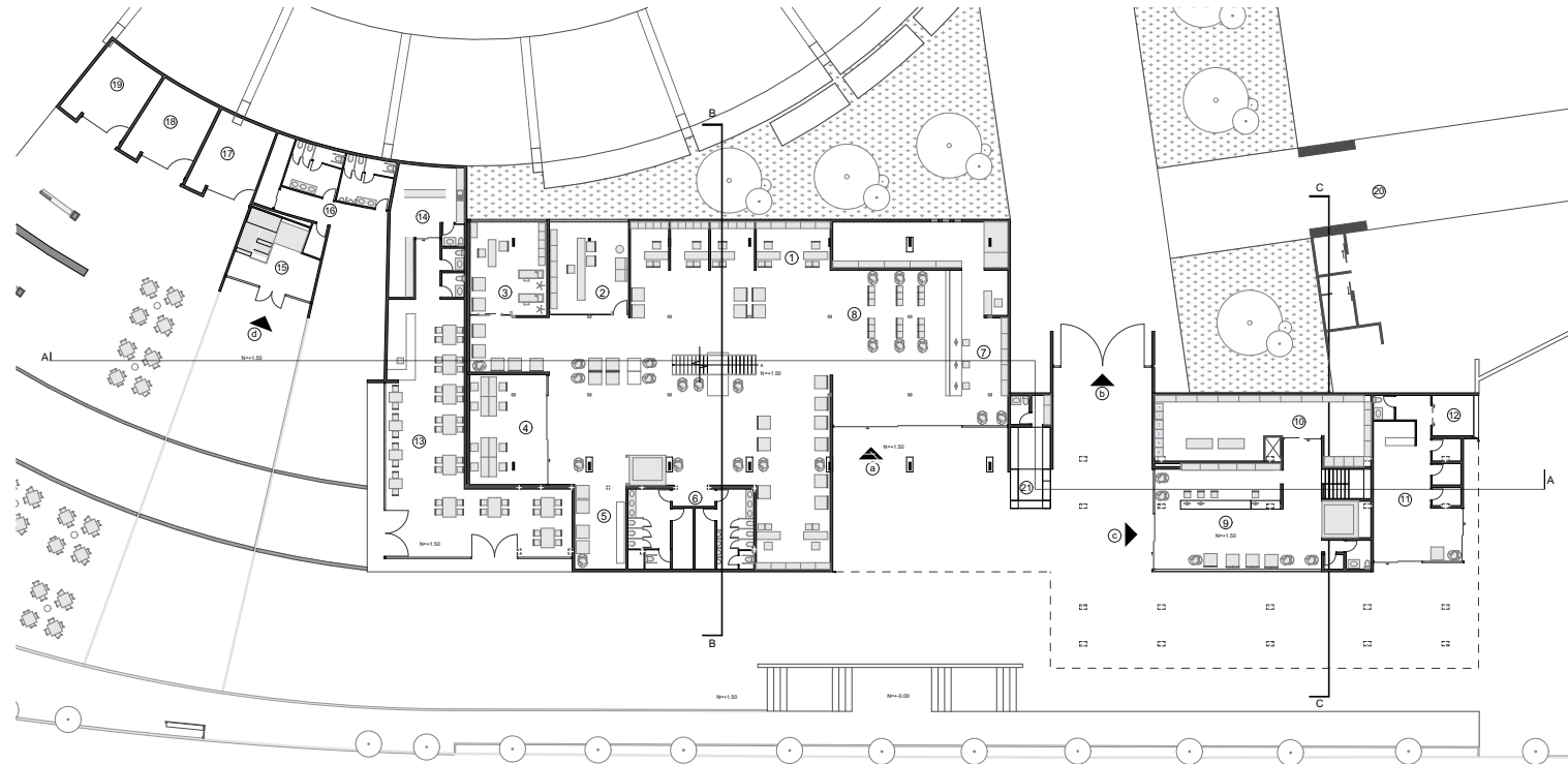
PLANTA BAJA
