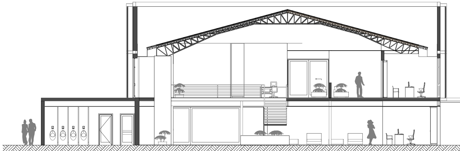
CORTE B-B 0 1 3 7
